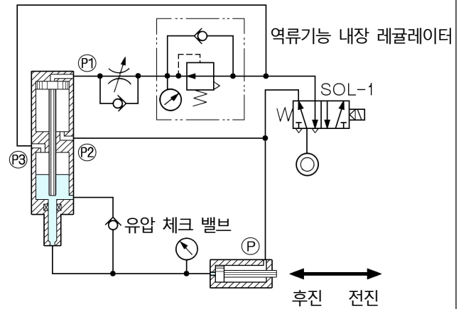
시작시 고추력 회로
